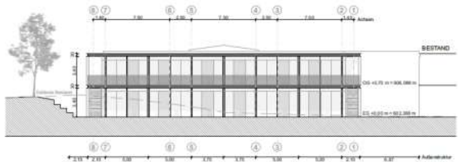
Ansicht Ost_M1_200
