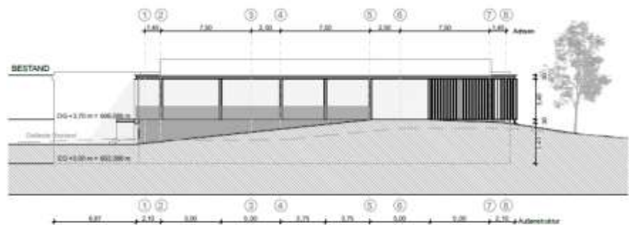
Ansicht West_M1_200
